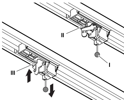
Fig. 18: Frigørelse og låsning af aktuator
