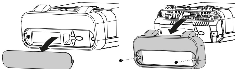
Fig. 9: Åbning af aktuatorhovedets dæksel
