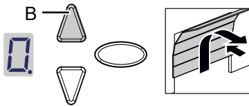
Fig. 16: Course d'apprentissage de l'effort
