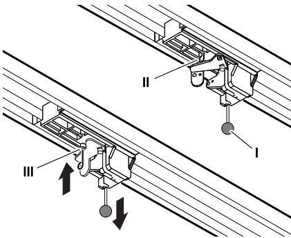
Afb. 18: Aandrijving ontgrendelen en vergrendelen
