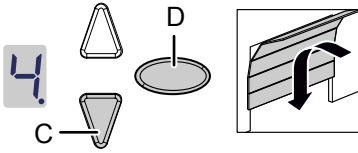
Abb. 15: Einstellung der Endposition ZU
