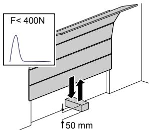
Fig. 17: Contrôle de la limitation d'effort
