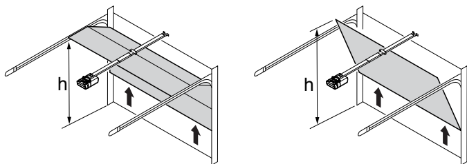
Fig. 7: Mesurer la hauteur totale de la porte de garage
