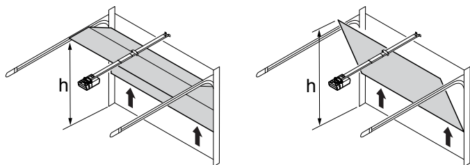
Fig. 7: Mål indvendig højde af garageporten
