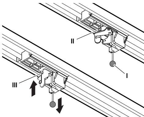
Fig. 18: Déverrouillage et verrouillage de l'entraînement
