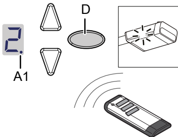
Abb. 12: Lichtfunktion für den Handsender programmieren
