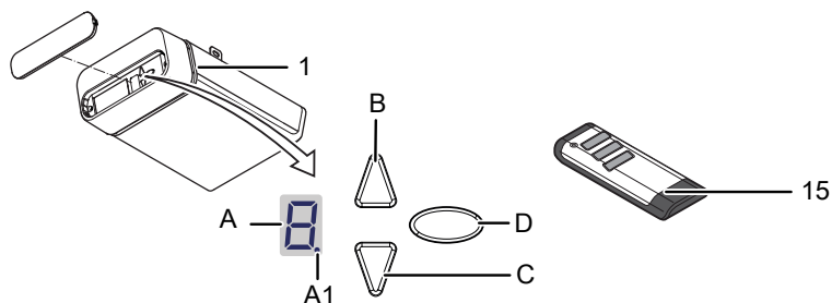
Fig. 4: Organes de commande
