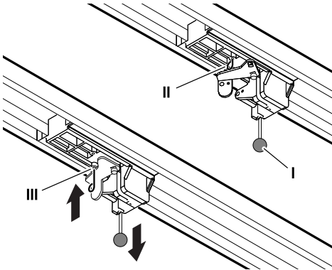
Abb. 18: Antrieb entriegeln und verriegeln
