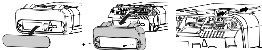
Fig. 10: Pose de l'antenne
