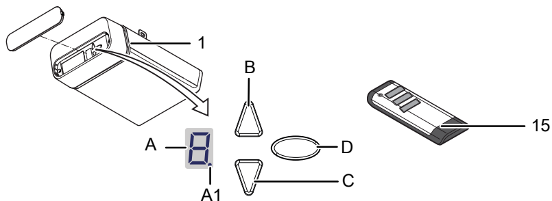
Afb. 4: Bedieningselementen
