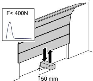
Afb. 17: Krachtbegrenzing controleren
