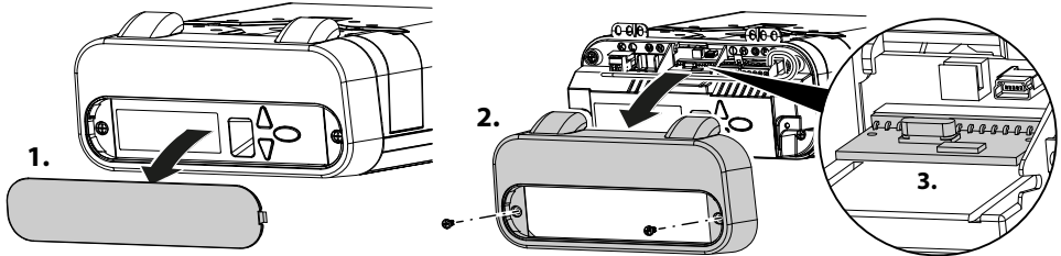
Abb. 2: Abdeckung am Antriebskopf öffnen und Funkmodul bestimmen
