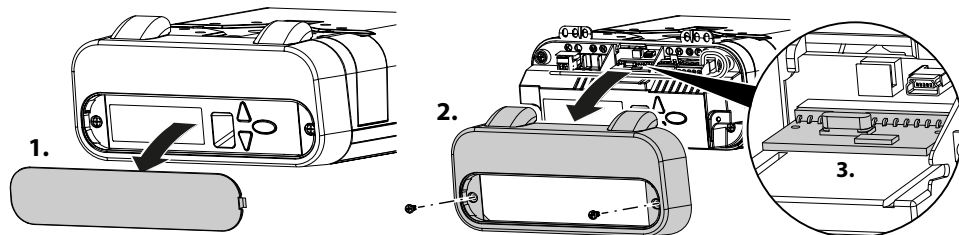
Fig. 2: Ôter le couvercle de la tête d'entraînement et déterminer le module radio
