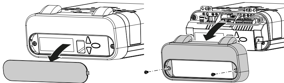
Fig. 9: Ouverture du couvercle de la tête de commande et d'entraînement
