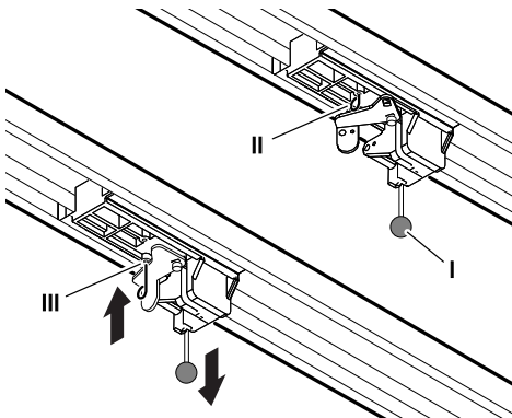
Abb. 8: Antrieb entriegeln und verriegeln
