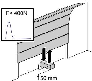
Abb. 17: Kraftbegrenzung prüfen
