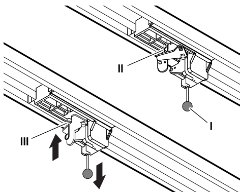
Fig. 8: Déverrouillage et verrouillage de l'entraînement
