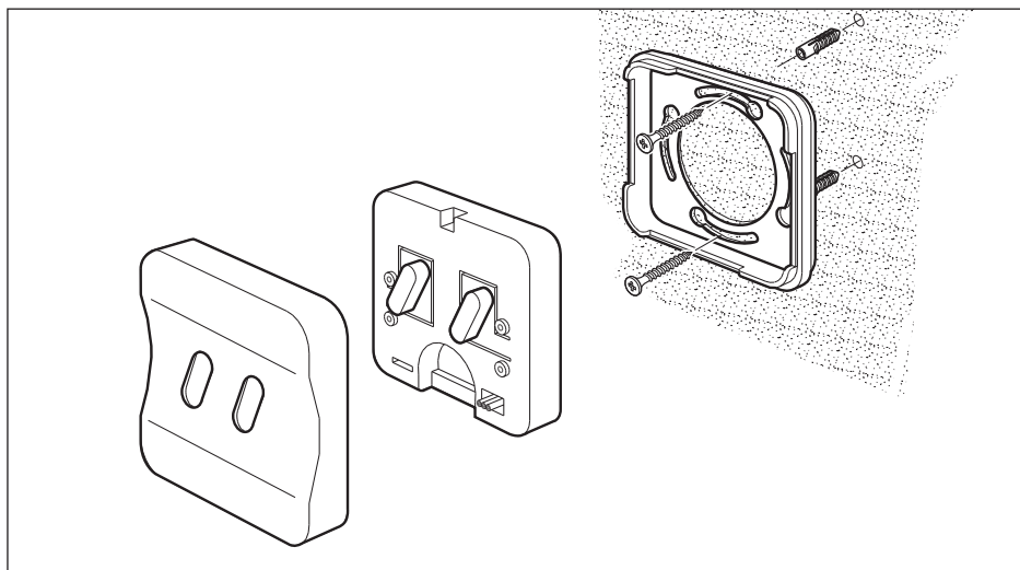
Afb. 3: Montage
