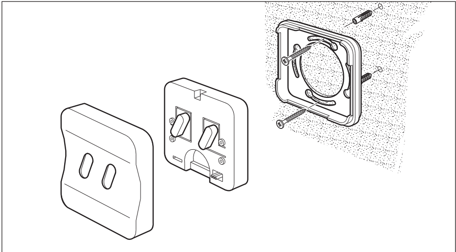
Abb. 3: Montage
